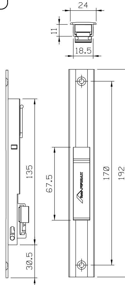
Vistas - escala 1:2
