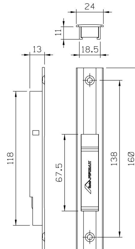
Vistas - escala 1:2
