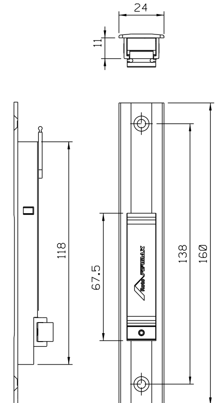
Vistas - escala 1:2
